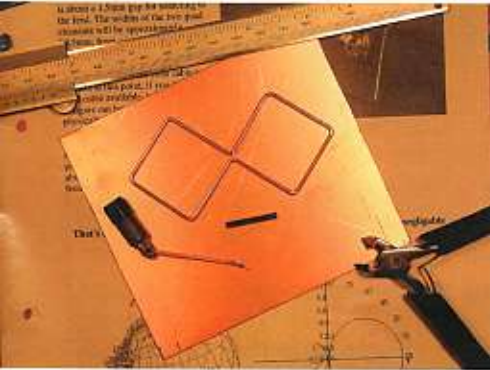
Biquad in voorbereiding. De straler bestaat uit een 244 mm lange draad, gebogen in 8 gelijke delen.
